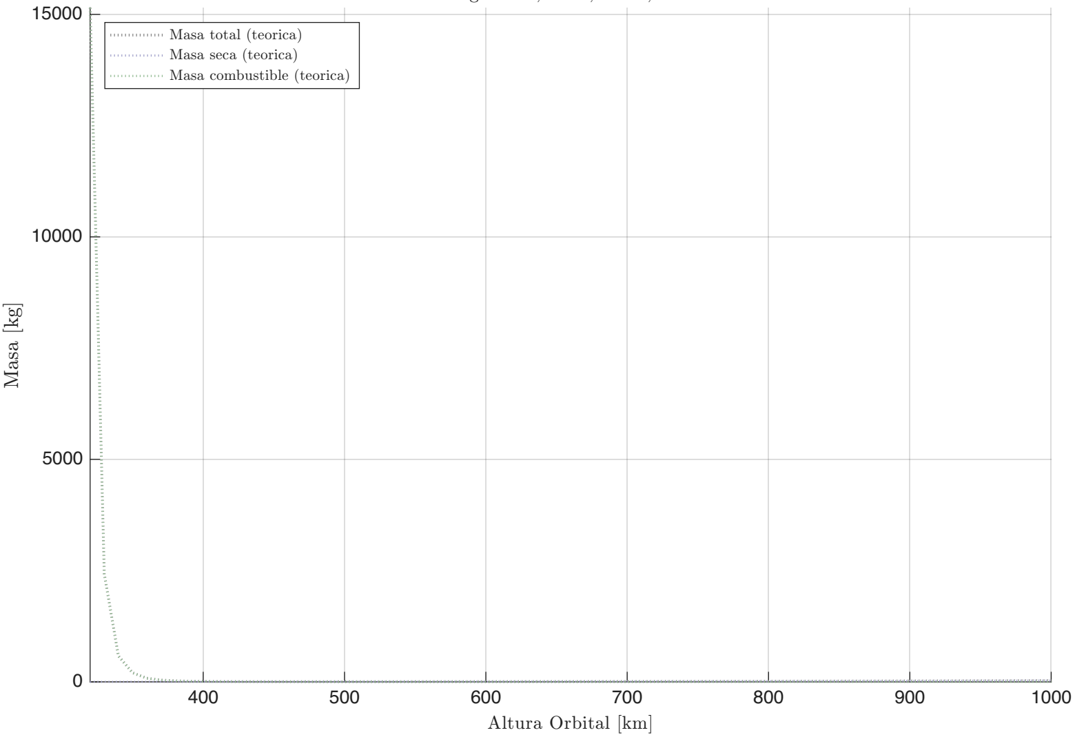
Desglose de Masas vs. Altura Config: 2 Sat, 2 Tel, Det 2, Korsch
